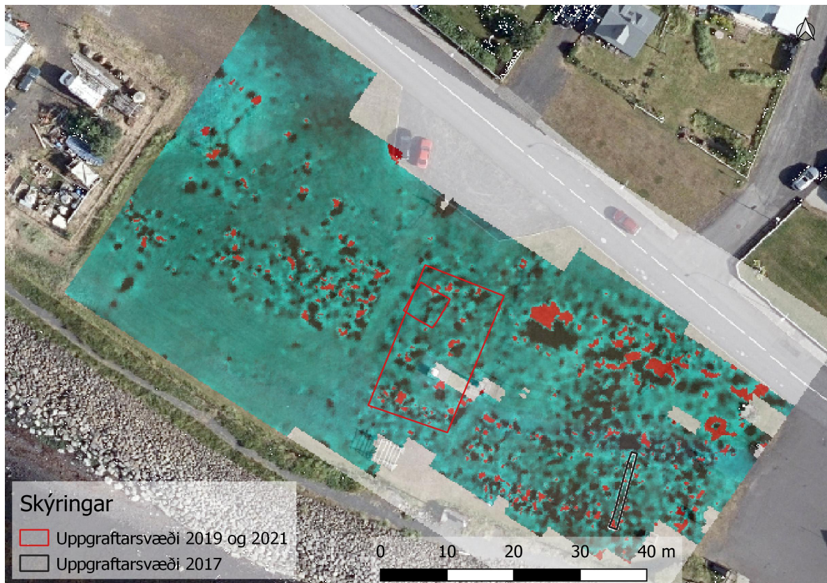
Mynd 3. Niðurstöður jarðsjármælinga sýna grjótundirstöður Vesturbúðarinnar. Grjótíð sést með rauðum og svörtum lit. Hvíta svæðið er hluti af veg sem var lagður eftir að húsin voru rifin. Kortið er gert af Mark Graham og Ragnheiði Gló Gylfadóttur.
