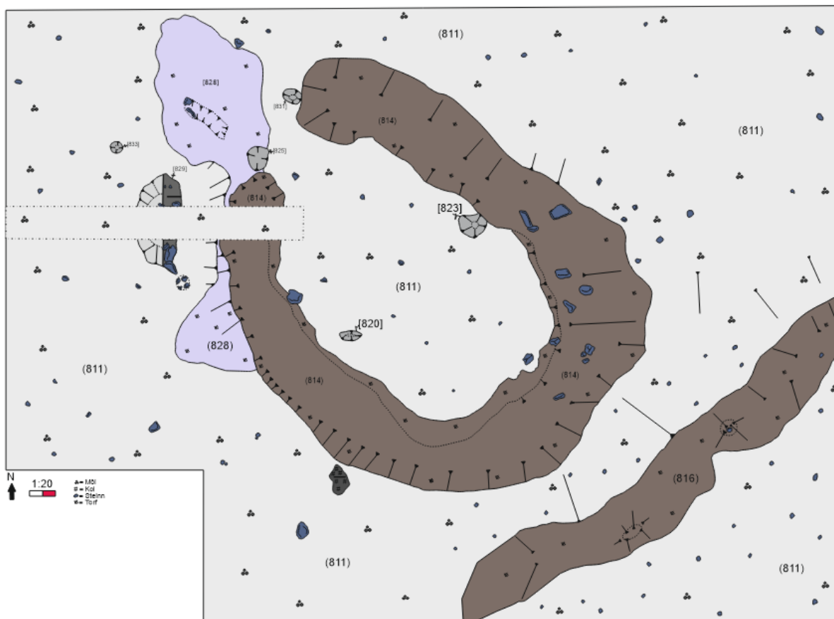
Mynd 41. Teikning í fleti af uppgriftarsvæði G við lok rannsókna. Tölvuteikning: Kristín Sylvía Ragnarsdóttir.
